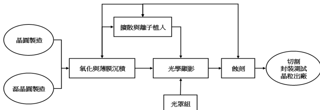
半導體製造流程圖
